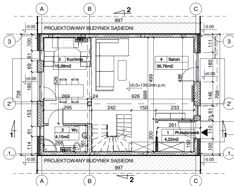
RZUT PARTERU
