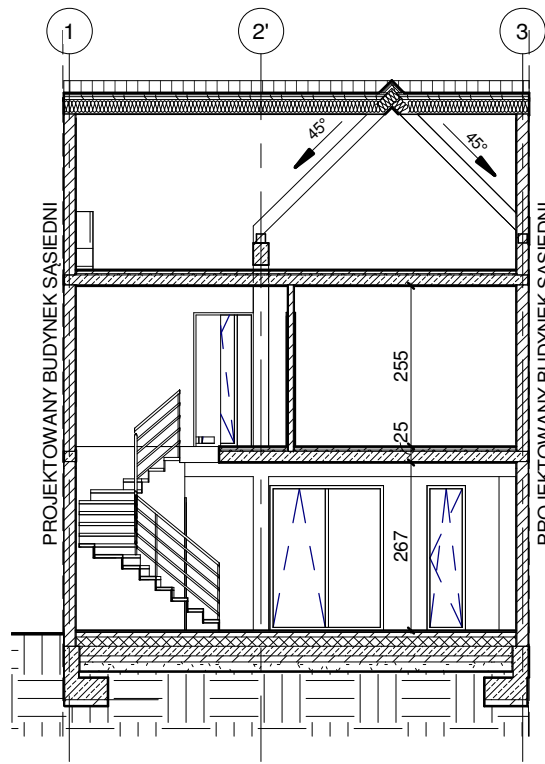
PRZEKRÓJ 2-2
