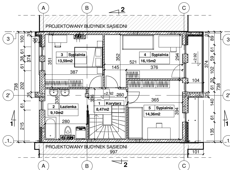
RZUT PIĘTRA
