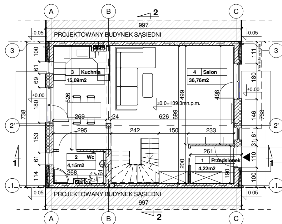
RZUT PARTERU
