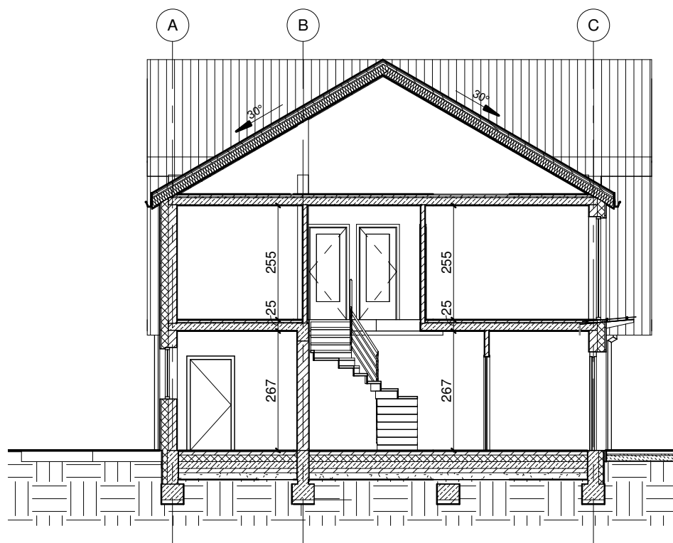
PRZEKRÓJ 1-1
